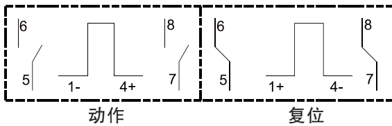
单线包(正接)
