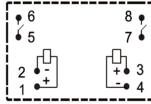
双线包(正接)
