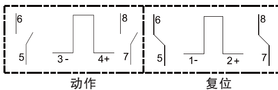
双线包(反接)
