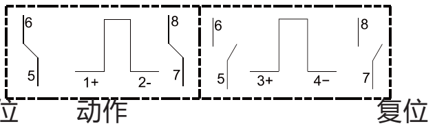
双线包(正接)
