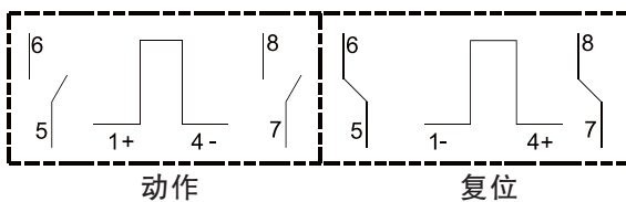
单线包(反接)
