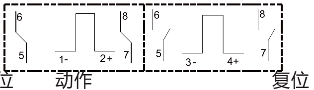
双线包(反接)
