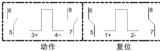
双线包(正接)
