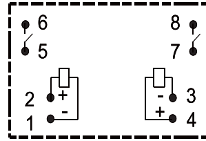
双线包(反接)
