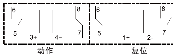
双线包(正接)
